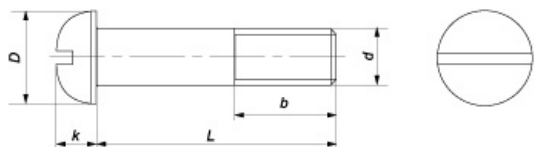
Исполнение 1 (прямой шлиц)
