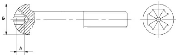
Исполнение 2 (крестообразный шлиц)
